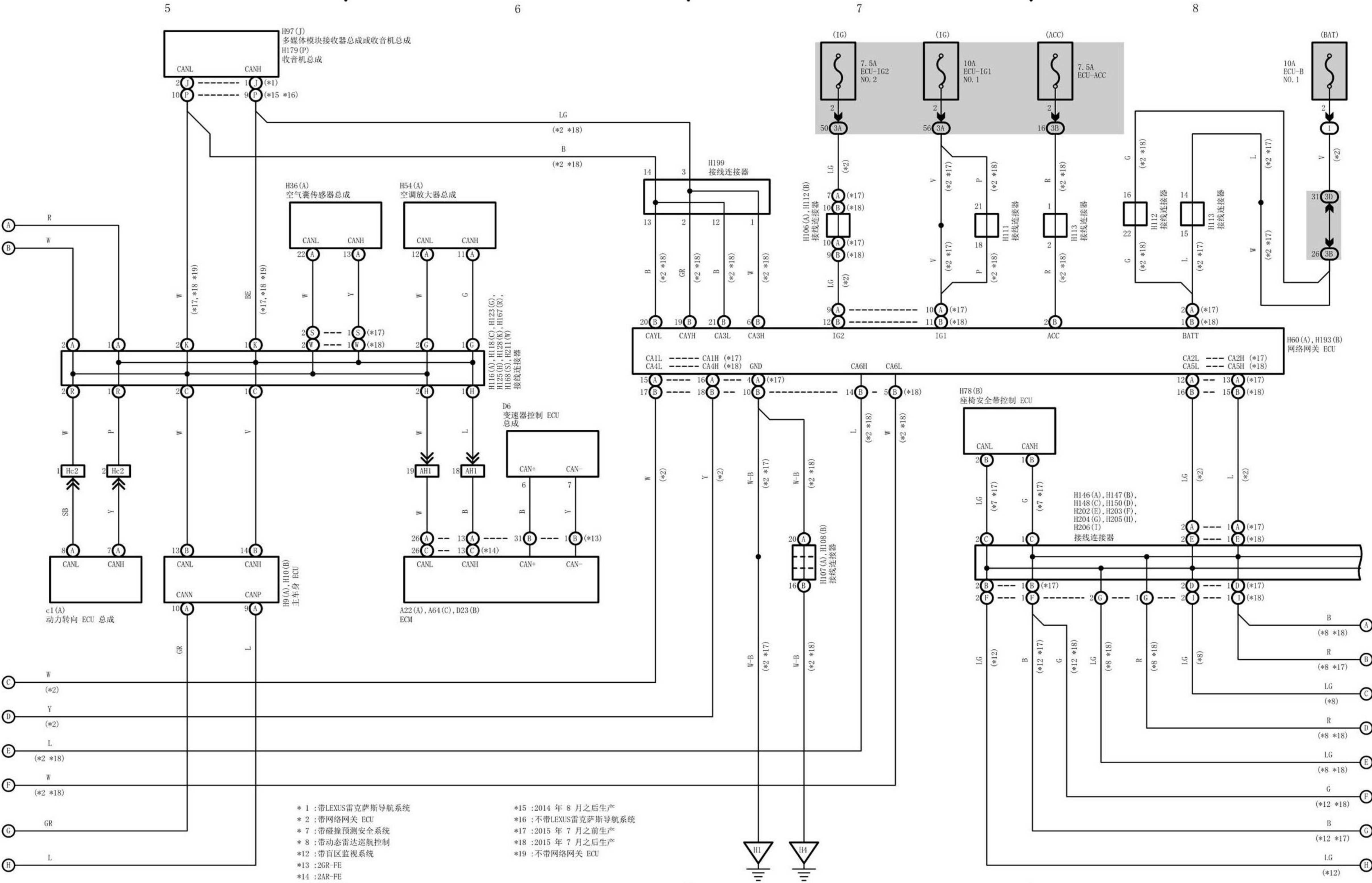
多路通信系统 (CAN) (右驾车型)
